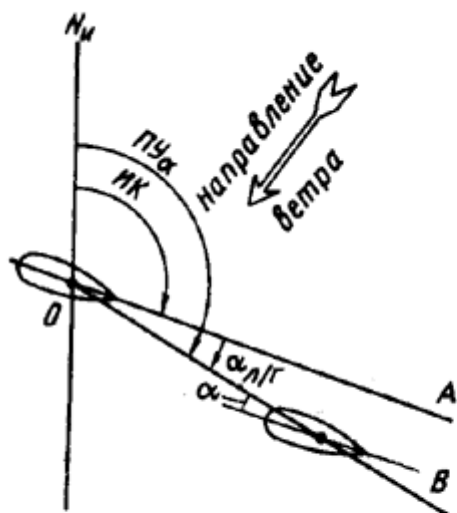
Рис. 33. Дрейф судна
