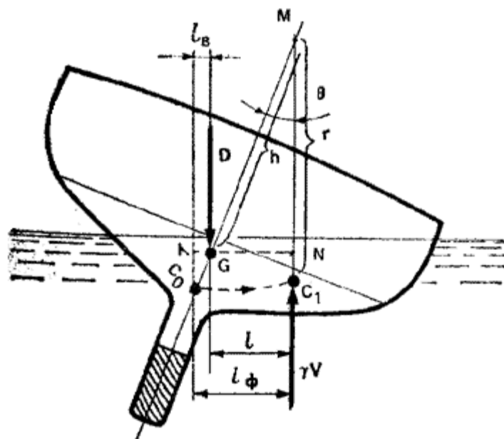
Остойчивость килевой яхты. Плечо остойчивости l = l_{\phi} - l_n
