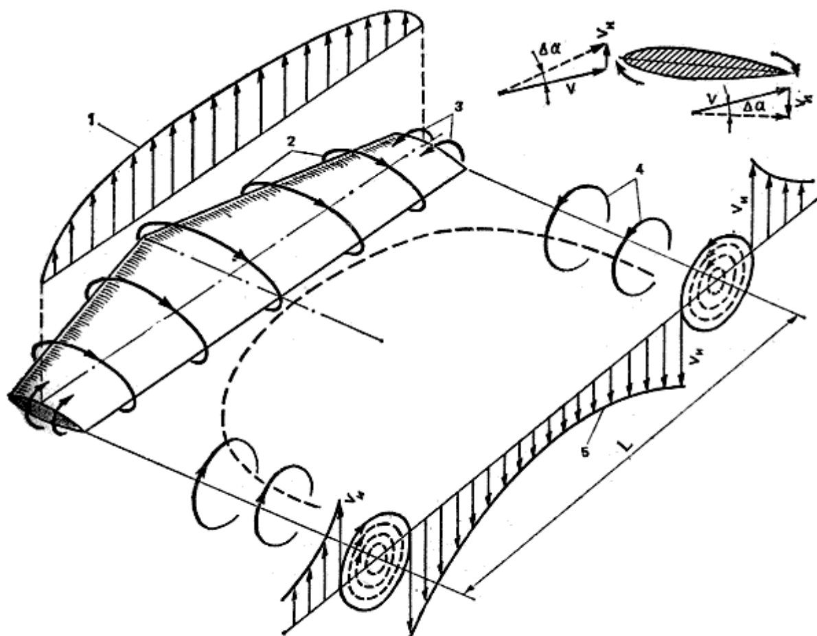
Рис. 10. Схема обтекания крыла конечного размаха:
