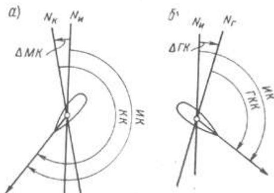
Рис. 16. Исправление курса
