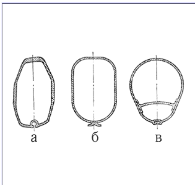
Рис. 39. Поперечное сечение мачт из легкого сплава:
