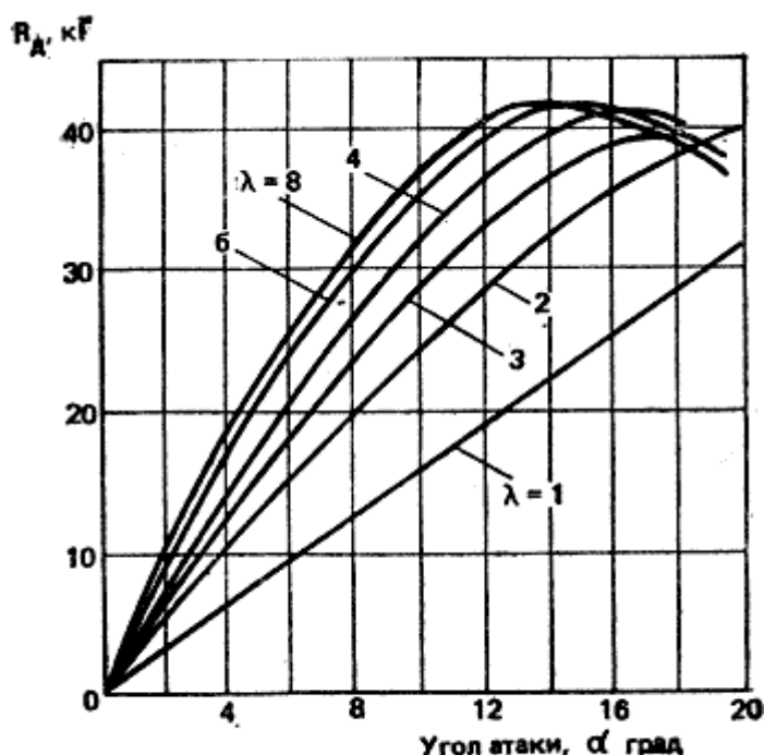
Рис. 11. Зависимость сопротивления дрейфу от удлинения киля и угла атаки
