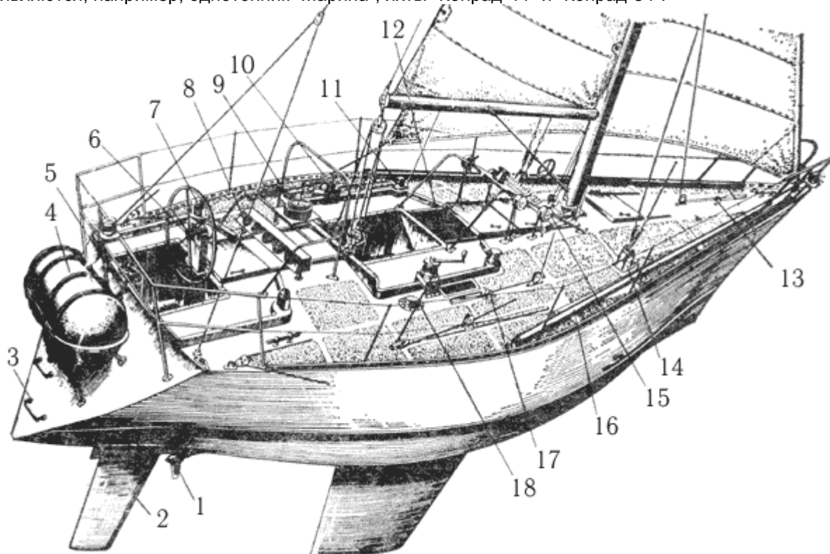
Рис. 32. Однотонок "Марина" постройки ленинградской судовой верфи ВЦСПС: 1 - гребной винт регулируемого шага; 2 - перо руля; 3 - скоб-трап; 4 - надувной спасательный плот ПСН-6М; 5 - привод натяжного ахтерштага; 6 - штурвал; 7 - путевой компас; 8 - приборная панель; 9 - главный компас; 10 - двухскоростная лебедка; 11 - односкоростная лебедка; 12 - входной люк; 13 - натяжка внутреннего штага; 14 - вант-путенс; 15 - фаловая лебедка; 16 - спинакер-гик; 17 - натяжка багштага; 18 - вентиляционный дефлектор.
