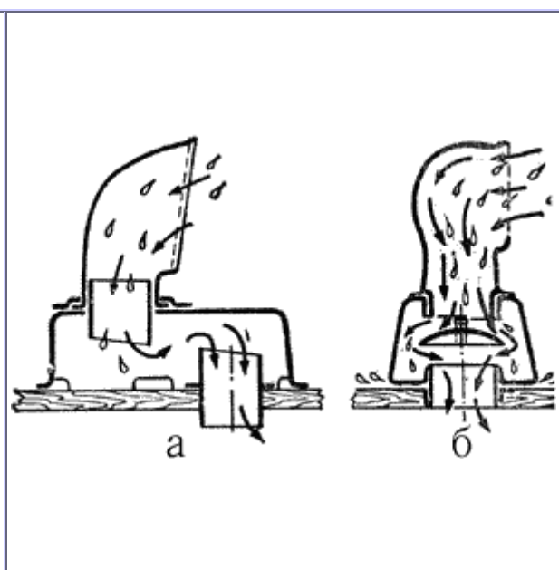
Рис. 38. Вентиляционные головки брызгозащищенного типа для яхт: а - типа "Дорадо"; б - фирмы "Никро Фико".
