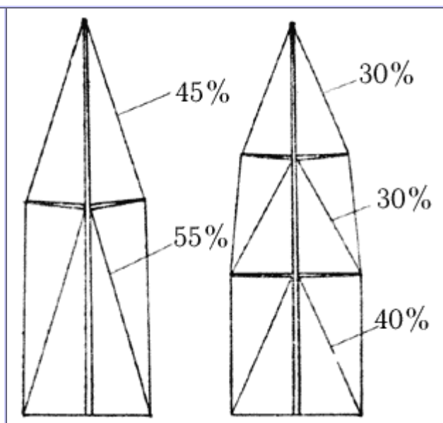
Рис. 40. Схема раскрепления мачт крейсерско-гоночных яхт и нагрузки на ванты в процентах от общего усилия.
