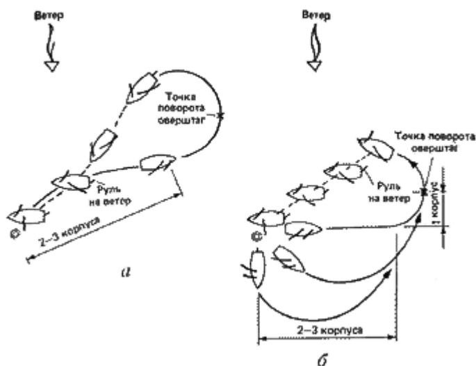
Рис.142: Подход к упавшему за борт с дрейфом: на курсе бейдевинд (а) и на курсах галфвинд, бакштаг и фордевинд (б).
