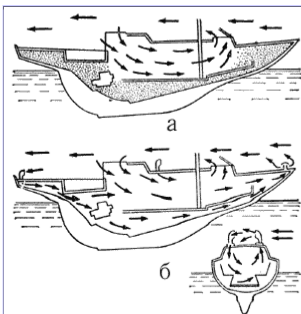
Рис. 37. Схема циркуляции воздуха в помещениях яхты. а - недостаточная циркуляция воздуха (заштрихованы неветилируемые объемы); б - правильная циркуляция воздуха.
