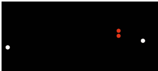
Вид ночью, судно длиной более 50 м
