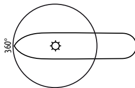
Возможная схема расположения огней при длине судна менее 50 м
