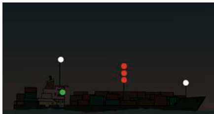
Вид с правого борта
