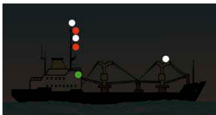
Вид с правого борта, имеет ход относительно воды
