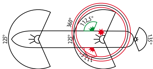
Схема расположения огней, имеет ход относительно воды
