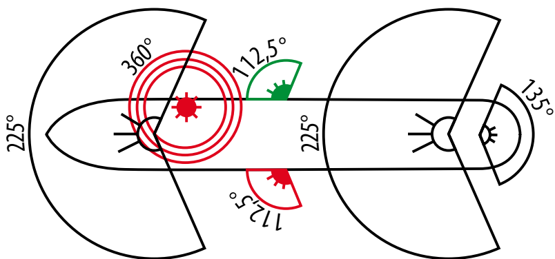
Схема расположения огней
