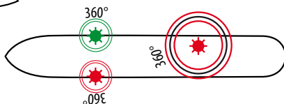
Схема расположения огней, на якоре
