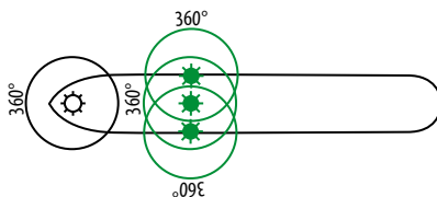
Схема расположения огней, на якорь
