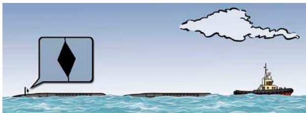
Вид днем при длине буксируемых объектов менее 200 м (правило 24 (g) (iv))
