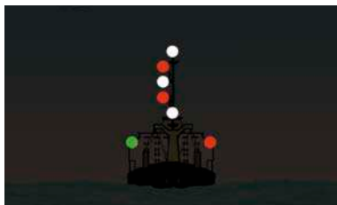
Вид с носа, имеет ход относительно воды
