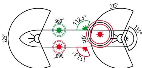
Схема расположения огней, имеет ход относительно воды
